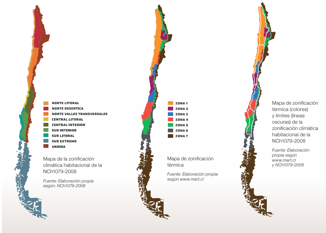
Figura 4.9. Mapas de zonificación térmica de Chile, según OGUC Art. 4.10
