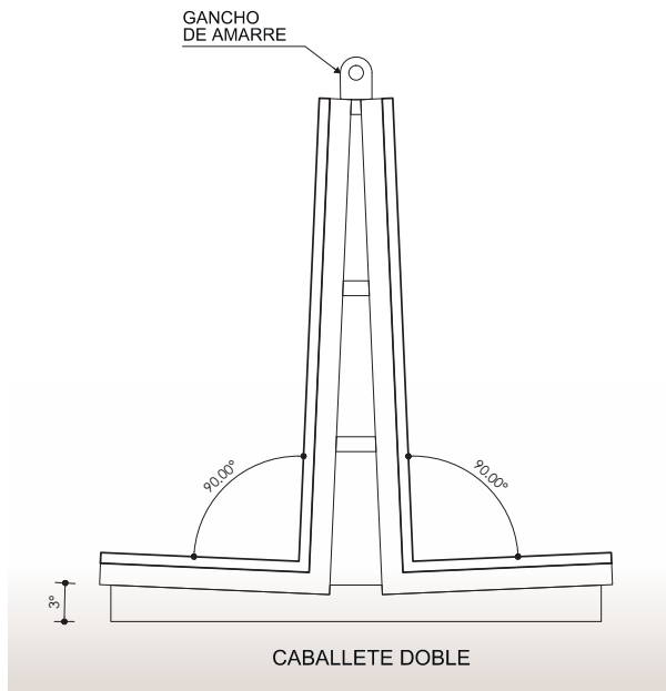
Figura 10.5. Atril de almacenamientos de paneles de muro cortina.
