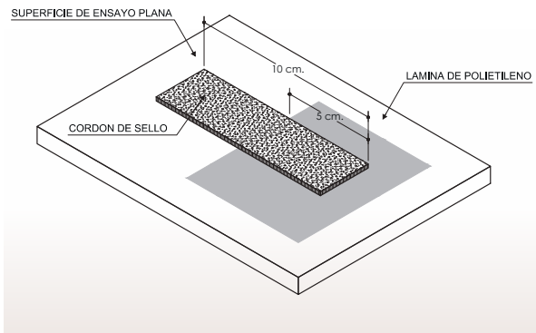
Figura 8.16. Probeta de ensayo de pelado de sello (peel-off) según norma ASTM C1401-02.
