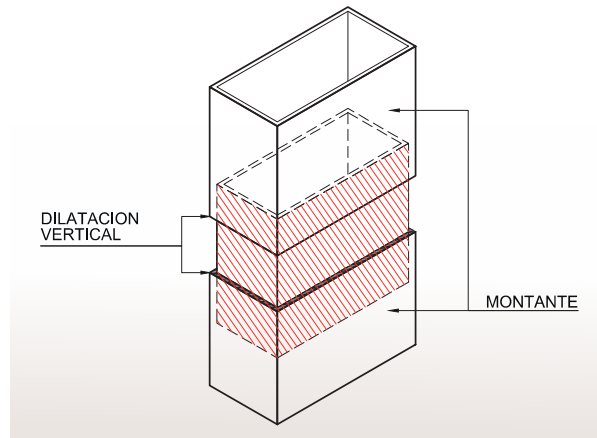
Figura 2.14. Deslizante de montante a montante.
