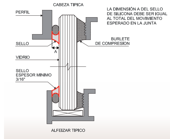
Figura 8.13. Recomendaciones para el sellado climático exterior.
