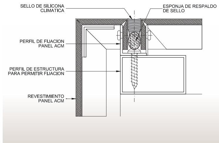
Figura 9.5. Detalle Horizontal de sellado de panel ACM (Con perfil ángulo de refuerzo en la esquina).
