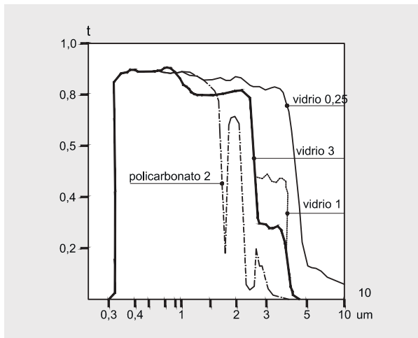
Figura 4.3. Transmisividad del vidrio y del policarbonato en función de la longitud de onda.
