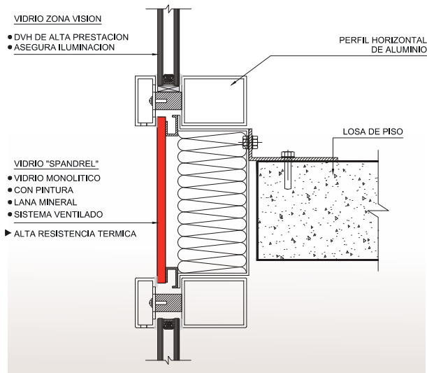
Figura 2.8. Muros cortina con vidrios de antepecho aislados térmicamente.
