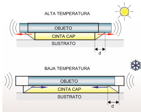
Figura 8.26. Dilatación y compresión de cinta CAP.
