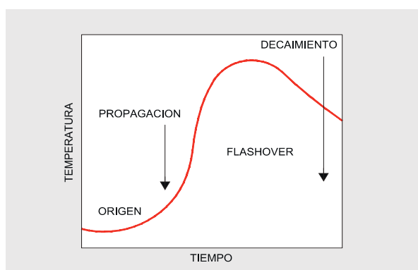
Figura 6.1. curva de evolución de la temperatura en un incendio en función del tiempo
