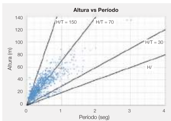
Figura 3.3. Distribución Altura Total Edificio respecto del periodo del primer modo traslacional (H/T).
