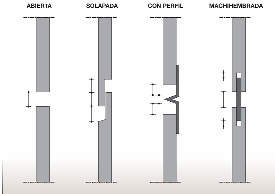
Figura 9.13. Sistemas de juntas de paneles de fachadas ventiladas.
