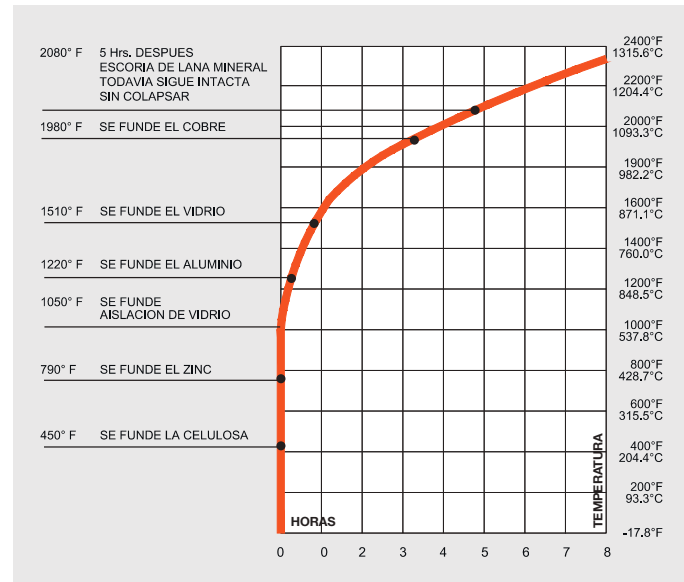
Figura 6.6. Curva tiempo - temperatura según ASTM E119.
