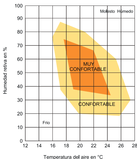
Figura 4.1. Gráfico de confort higrotérmico.
