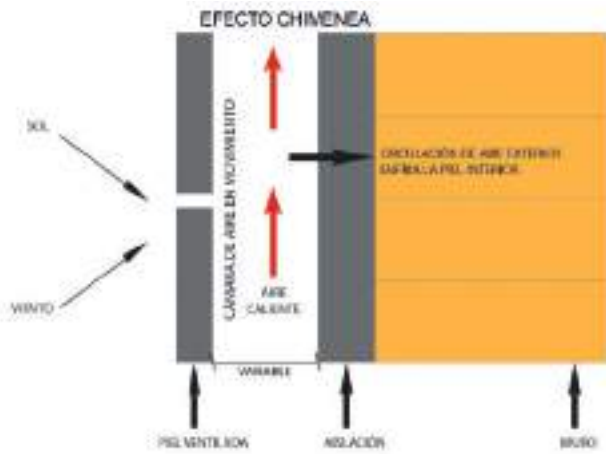
Figura 9.8. Principio de funcionamiento de fachadas ventiladas.
