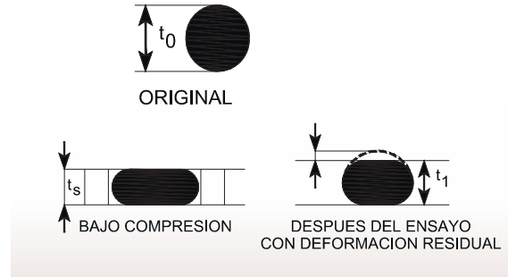
Figura 8.20. Deformación por compresión de un burlete.
