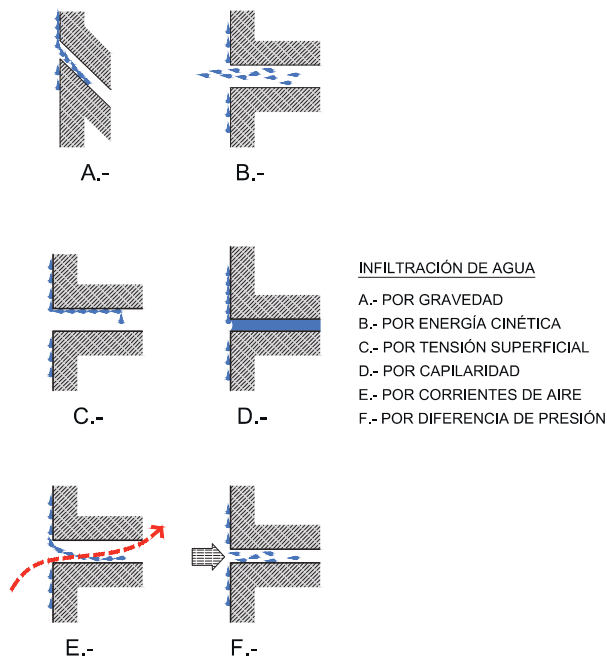
Figura 2.2. Causas de infiltración de agua.
