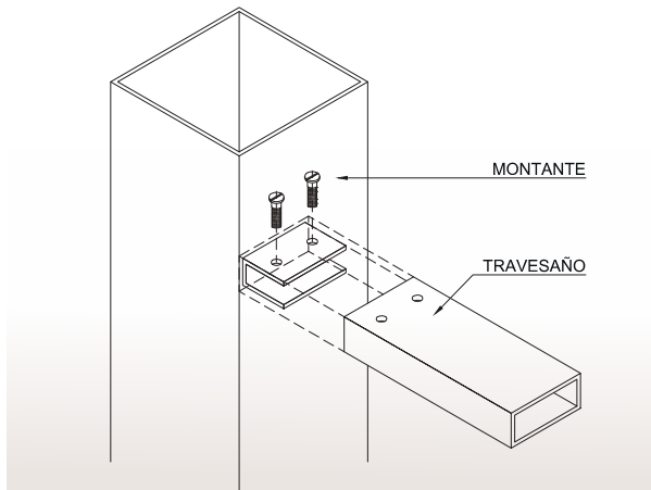
Figura 2.13. Unión fija de travesaño a montante.
