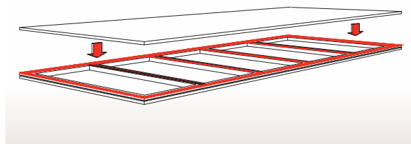
Figura 8.28. Aplicación de cinta CAP para panel arquitectónico.
