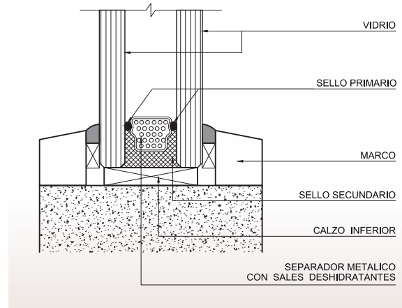
Figura 4.14. Detalle de ventana marco perimetral.
