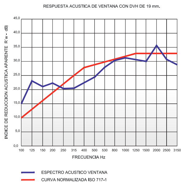
Figura 2.9. Espectro de respuesta acústica de ventana con DVH de 19 mm.
