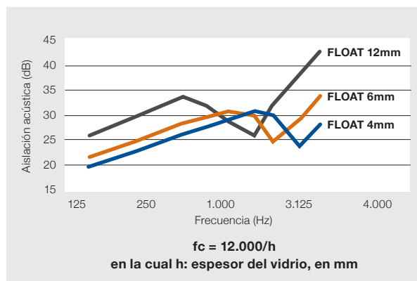
Figura 5.6. Nivel de Aislación Acústica (dB) de un cristal flotado en función de la frecuencia (Hz).
