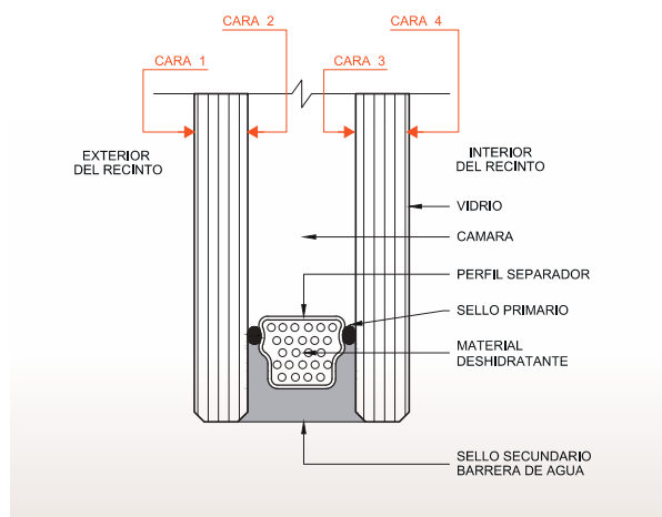
Figura 8.7. Esquema de un doble vidrio hermético.
