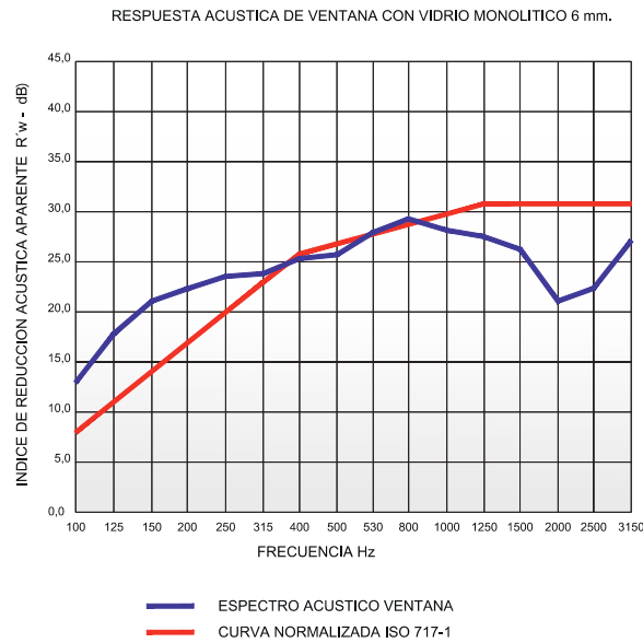
Figura 2.10. Espectro de respuesta acústica de ventana con vidrio simple de 6mm.
