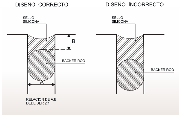
Figura 8.9. Recomendaciones de diseño de juntas.
