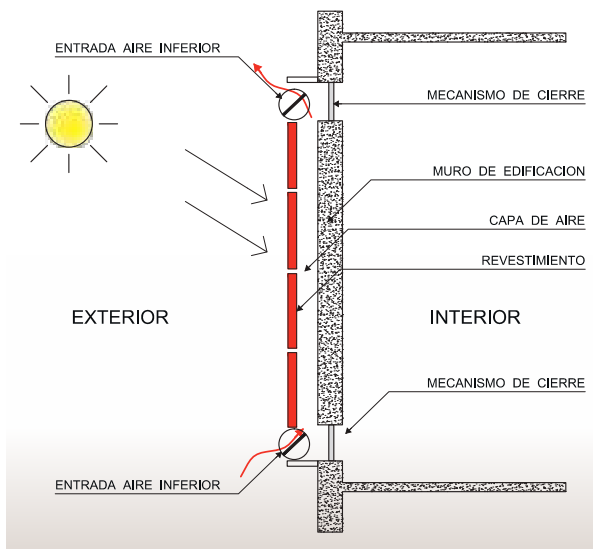
Figura 9.11. Detalle de cámara de aire de fachada ventilada.
