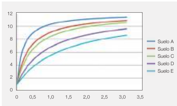
Figura 3.4. Factor de modificación de respuesta R^* según tipología de suelos del DS61 (en el gráfico se ha considerado R_0=11 ).
