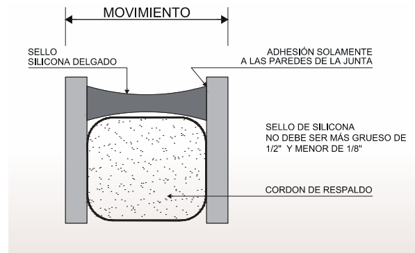
Figura 8.10. Detalle de junta con sello y cordón de respaldo.
