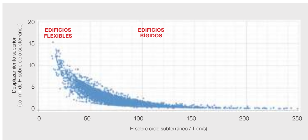
Figura 3.13. Desplazamiento de nivel superior en función de la rigidez (H/T).
