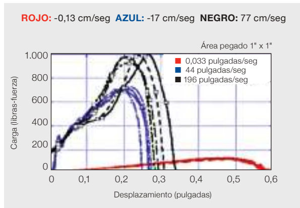
Figura 3.12. Curva tensión deformación de cinta acrílica CAP sometida a diferentes velocidades de aplicación de carga dinámica.
