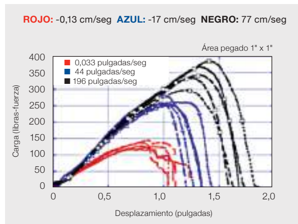
Figura 3.10. Curva tensión deformación de silicona estructural sometida a diferentes velocidades de aplicación de carga dinámica.
