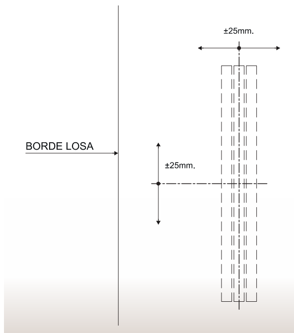
Figura 10.3. Esquema referencial de insertos con tolerancias en el hormigón (Losa e insertos).
