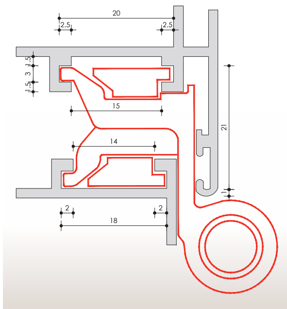
Figura 9.7. Detalle de perfil de aluminio con "cámara europea".
