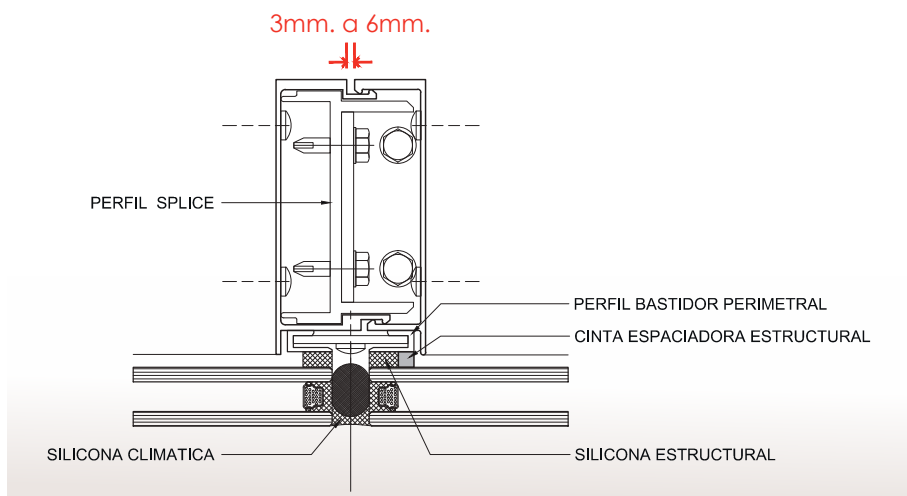
Figura 3.7. Splice conectada al mullion macho.
