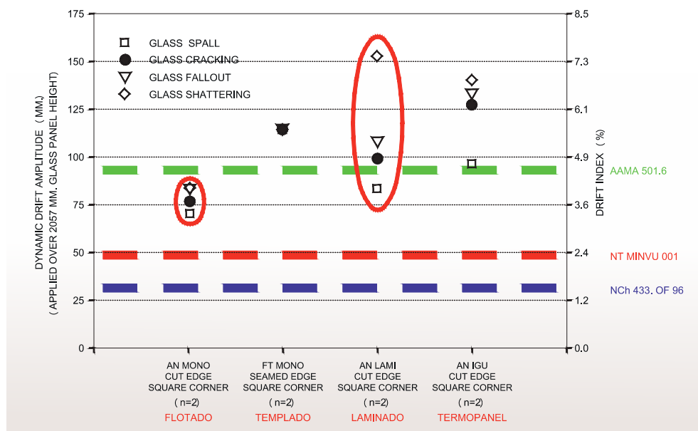
Figura 3.8. Ensayos de absorción de deformación de entrepiso de paneles con silicona a ambos lados.
