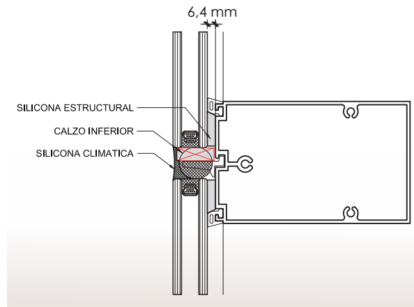
Figura 3.9. Detalle típico de muro cortina con silicona estructural cuatro lados, con DVH y calzo inferior.
