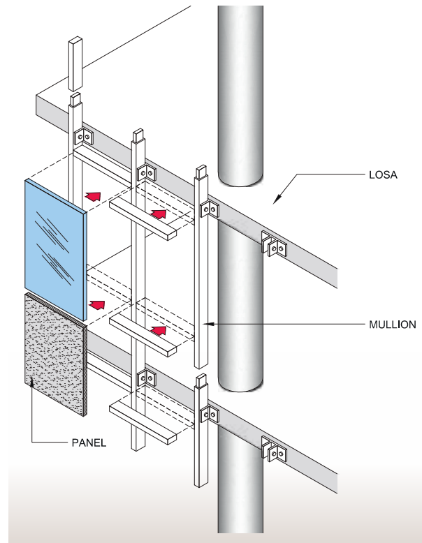
Figura 10.8. Secuencia de instalación de muro cortina con sistema stick.
