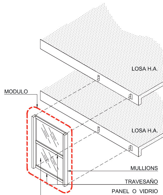
Figura 1.4. Sistema de Muro Cortina Tipo Frame.
