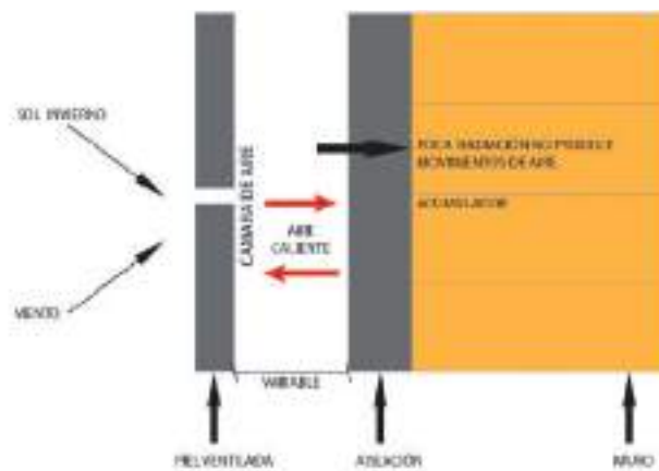
FACHADA VENTILADA INVIERNO
