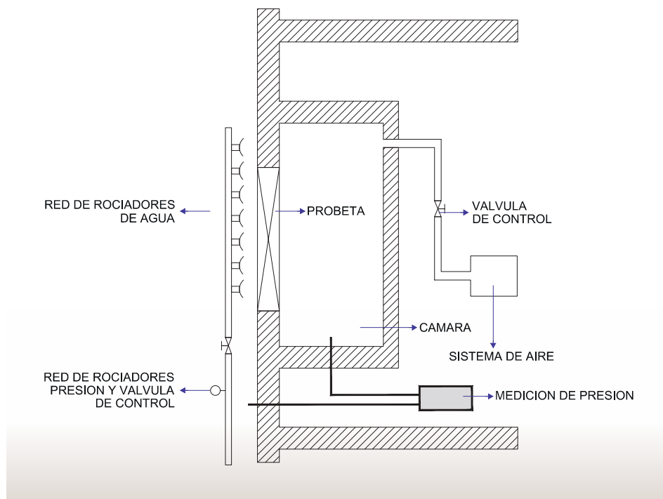
Figura 11.1. Ensayo de penetración del agua, según norma NCh 2808.Of2003.
