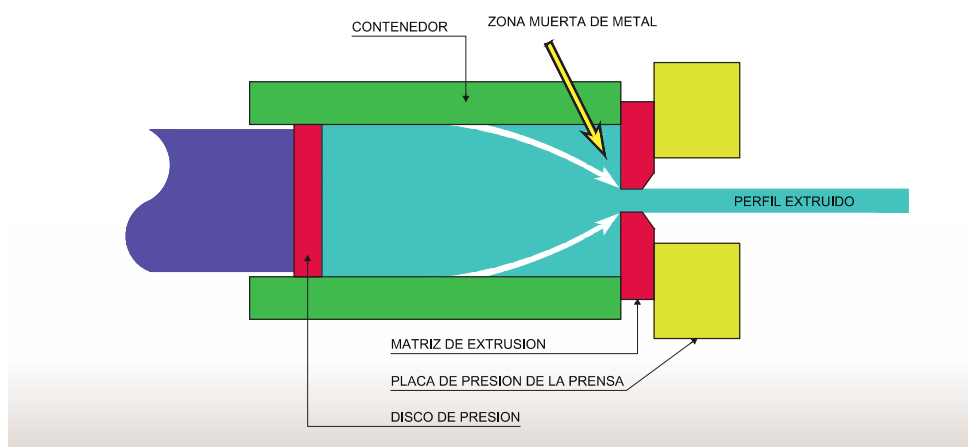
Figura 9.1. Tocho de aluminio a la salida de la prensa de extrusión
