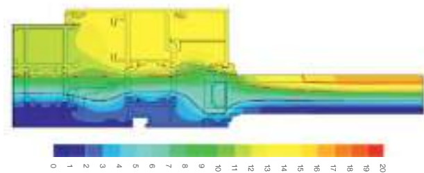
Figura 4.15. Variación de temperatura de una superficie vidriada con marco perimetral.
