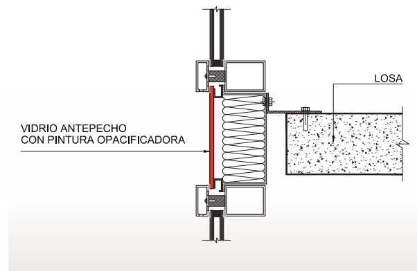
Figura 4.17. Detalle de vidrio de antepecho opacificado, frente a la losa de piso.
