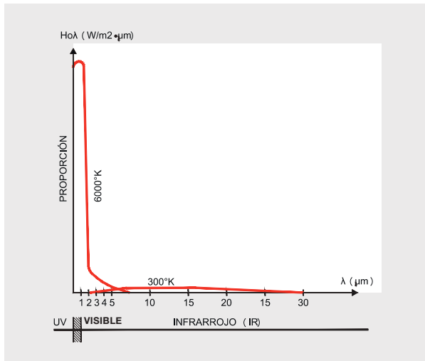
Figura 4.2. Radiación emitida por los cuerpos en función de la longitud de onda.
