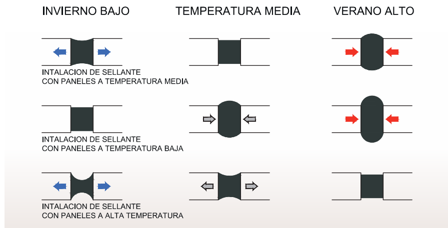
Figura 8.11. Efecto de la temperatura en la aplicación del sello de junta
