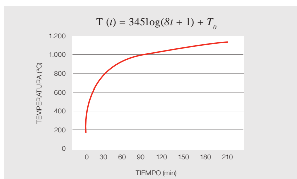
Figura 6.2. curva estándar de desarrollo de temperatura en función del tiempo.
