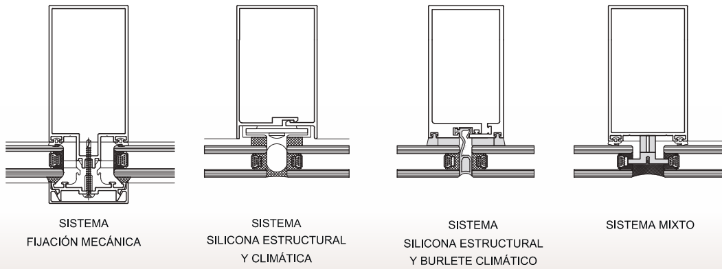
Figura 4.18. Diferentes sistemas de fijación de muros cortina.
