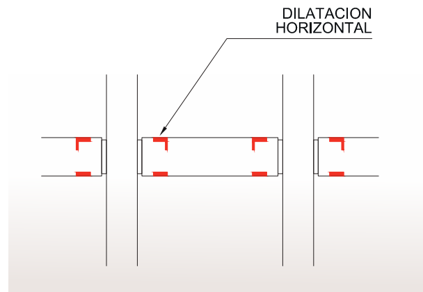
Figura 2.12. Dilatación horizontal de travesaños.
