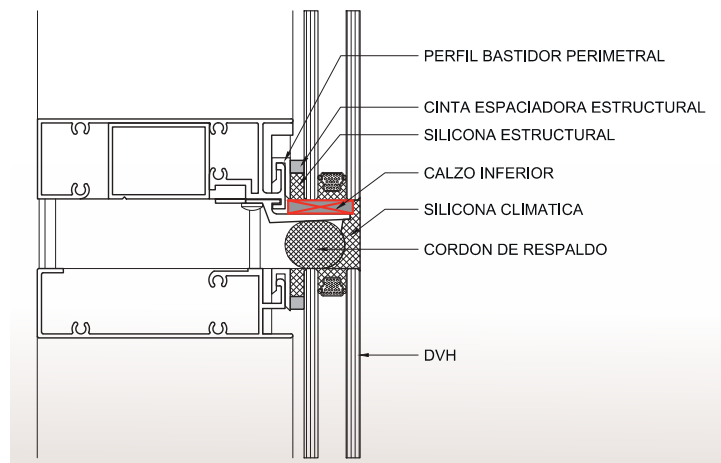
Figura 3.6. Calzos Inferiores.
