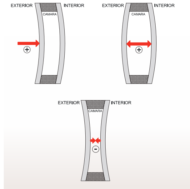
Figura 8.8. Efectos de las presiones positivas y negativas en un DVH.
