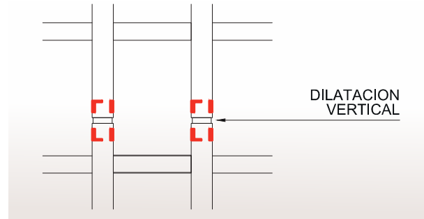
Figura 2.11. Dilatación vertical de mullions.
