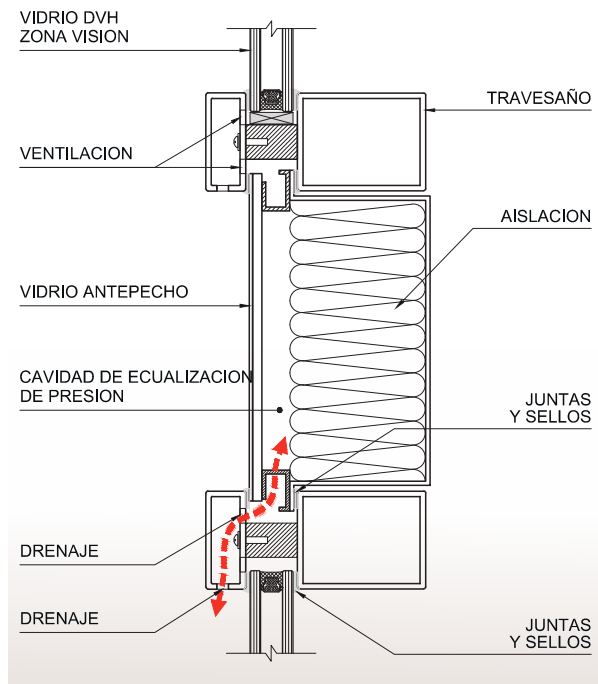
Figura 2.7. Sistema de muro cortina con ecualización de presiones.
