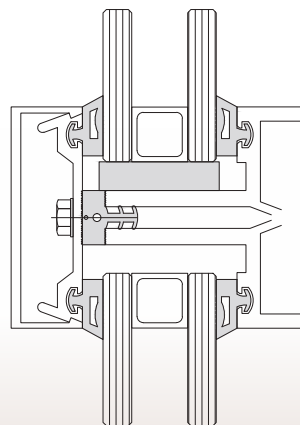
Figura 8.22. Detalle muro cortina con tapa presora burleteada.
