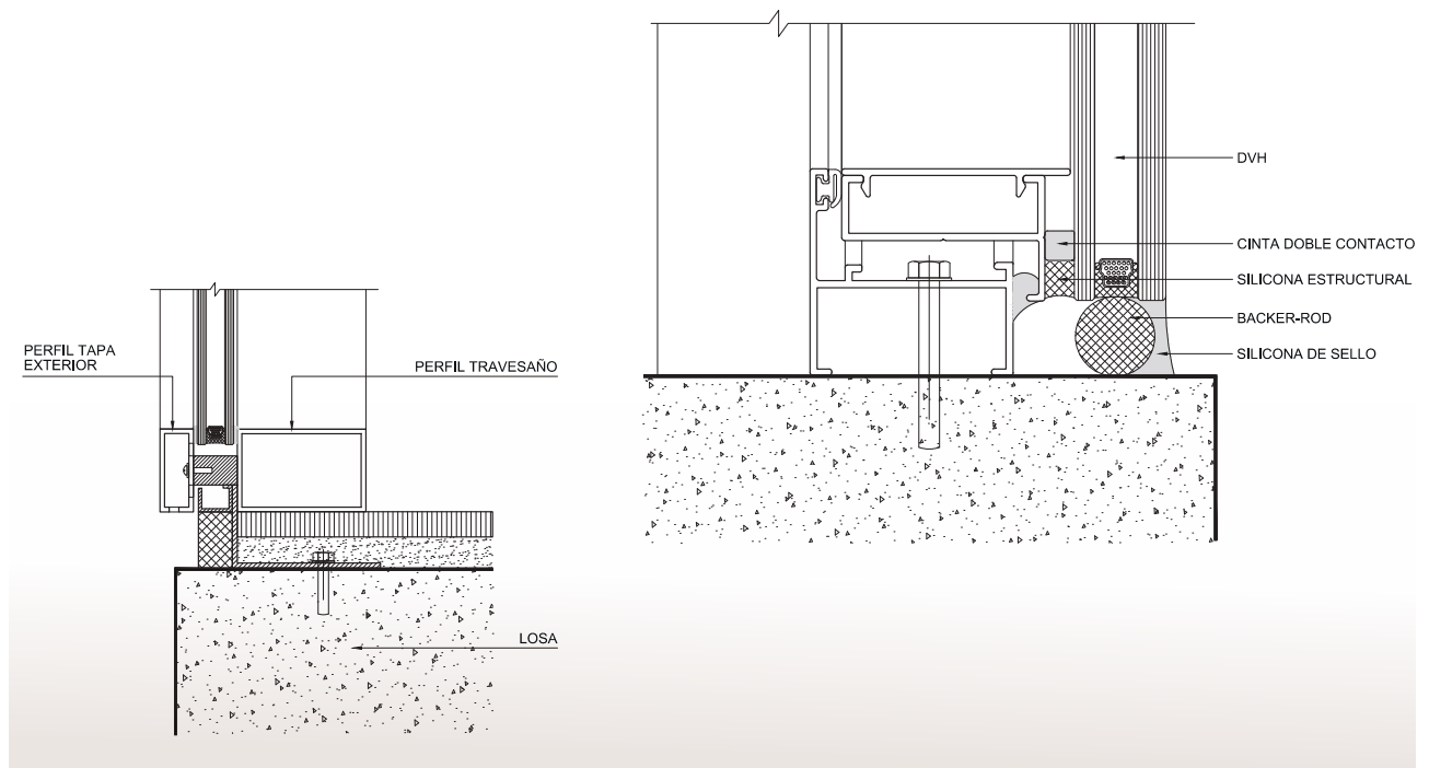
Figura 2.16. Remate arranque inferior.
