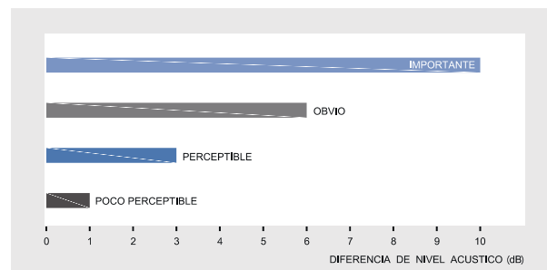
Figura 5.4. Perceptibilidad de los niveles acústicos.
