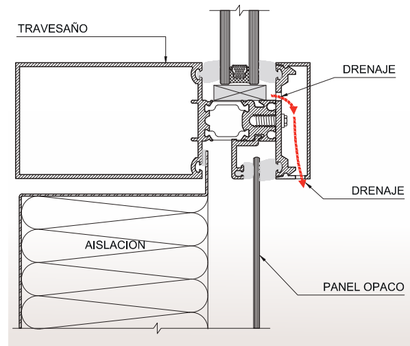
Figura 2.6. Sistema de drenaje de aguas lluvias de muro cortina.
