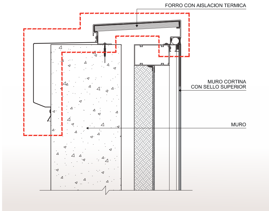
Figura 2.15. Remate exterior de coronación.
