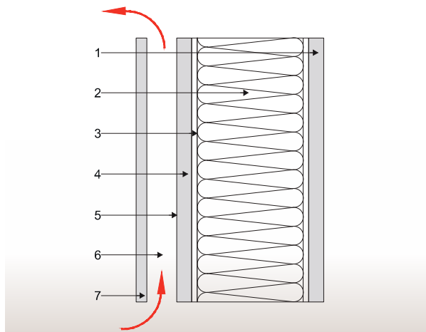
Figura 9.10. Cerramiento con hoja interior de obra seca.
