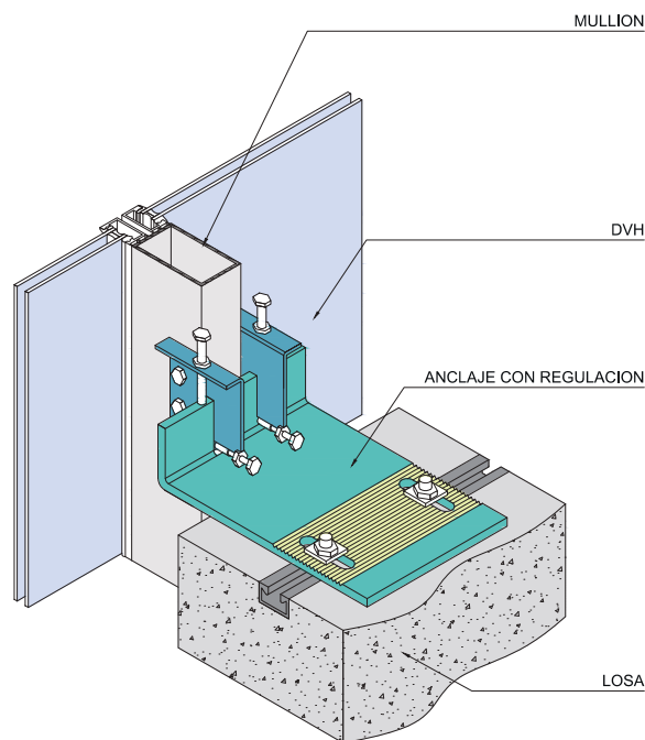
Figura 1.5. Sistema de anclaje del muro cortina a losa.
