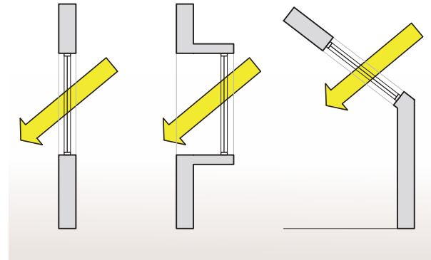
Figura 2.1. Ganancias de radiación solar en diferentes soluciones arquitectónicas.
