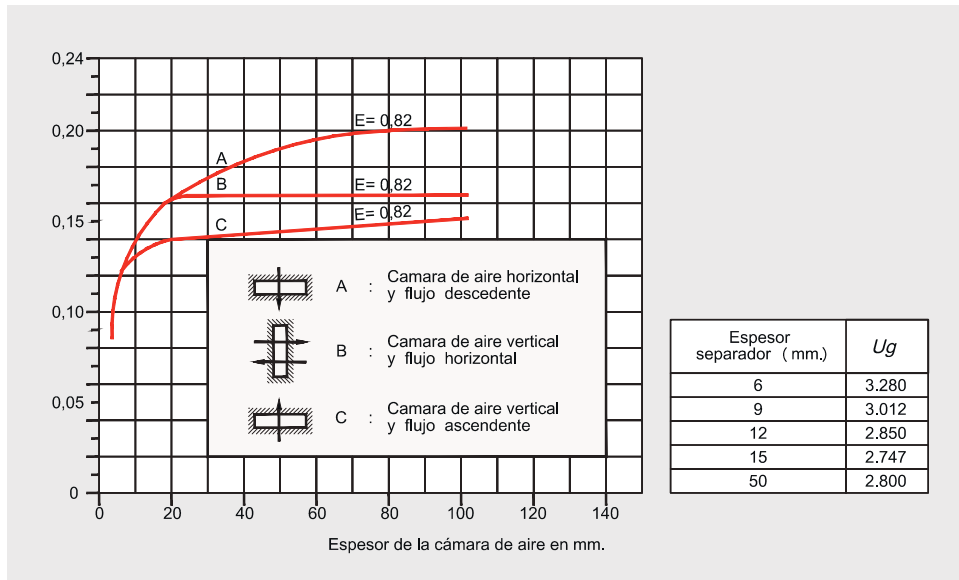
Figura 4.16. Resistencia térmica de cámaras verticales no ventiladas según NCh 853Of.91
