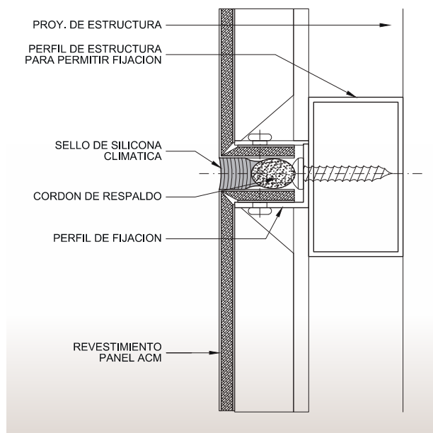
Figura 9.4. Detalle Vertical de sellado de panel ACM.
