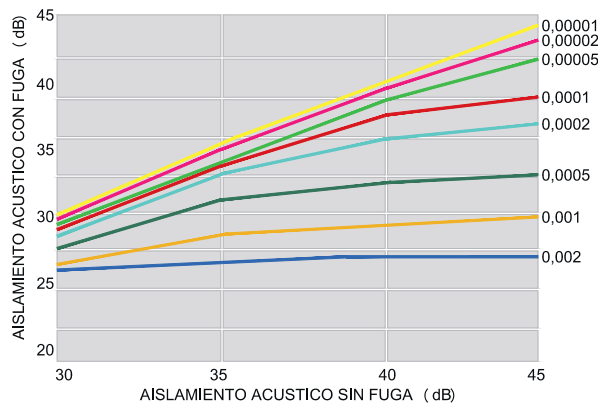
Figura 5.9. Disminución de aislamiento acústico en función del área de fuga.
