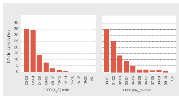
Figura 3.1. Máximo desplazamiento de entrepiso en C. de G.
