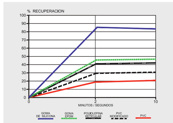
Figura 8.21. Recuperación (en minutos) de la geometría de diferentes materiales empleados en la producción de burletes, con probetas plegadas en un ángulo de 0°, con un envejecimiento térmico a 50°C durante 70 horas.
