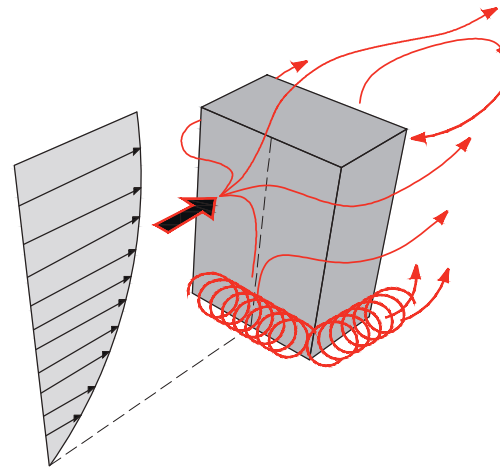
Figura 2.3. Diferencias de presión producidas por el viento.
