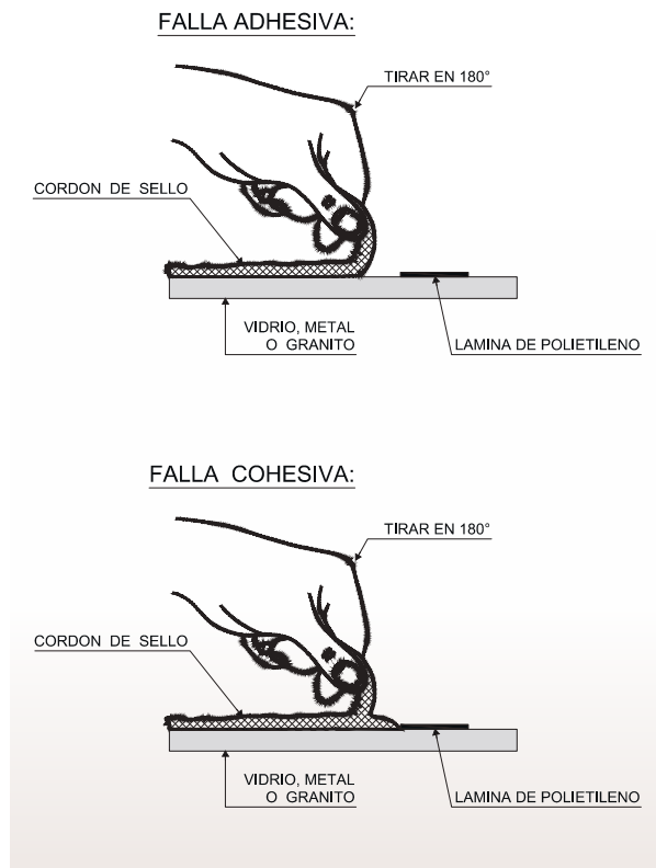
Figura 8.17. Ensayo de pelado de sello (peel-off) según norma ASTM C1401-02.
