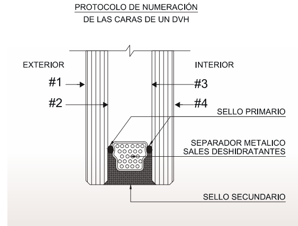
Figura 4.13. Protocolo de numeración de las caras de un DVH.
