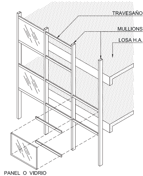
Figura 1.3. Sistema de Muro Cortina Tipo Stick.
