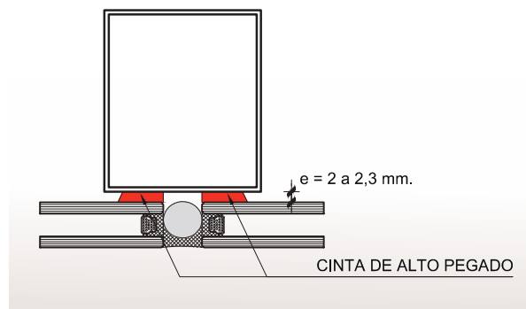
Figura 3.11. Detalle típico de panel vidriado con cinta de alto pegado (CAP) (Ver capítulo 8).
