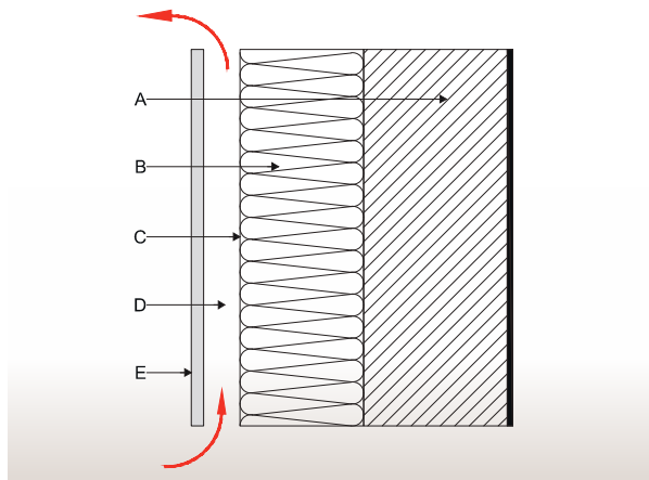
Figura 9.9. Cerramiento con hoja interior de obra húmeda.
