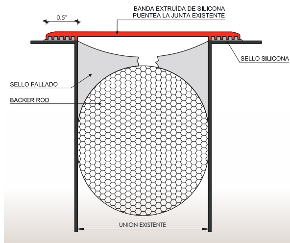
Figura 14.5. banda de silicona para reparar junta dañada.
