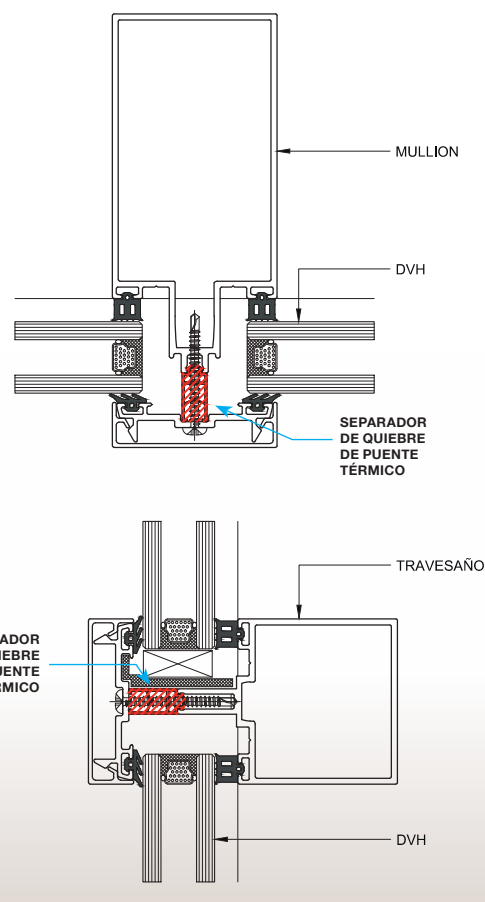
Figura 9.2. Detalle de perfil de aluminio con varilla de rotura de puente térmico.
