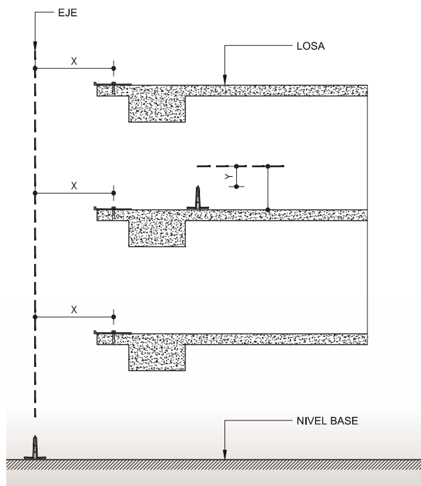
Figura 10.2. Sección vertical que muestra ejes de instalación.
