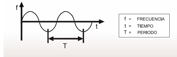
Figura 5.2. Periodo de una onda sonora.
