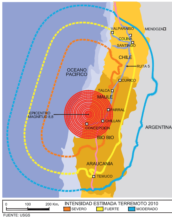
Figura 2.4. Intensidades estimadas del terremoto de Chile 2010
