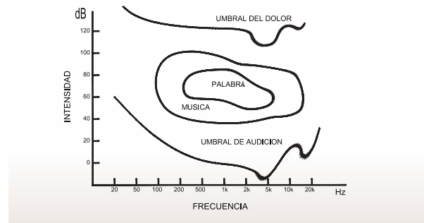
Figura 5.3. Intensidad de la onda sonora (dB) en función de la frecuencia (Hz).
