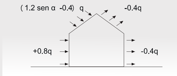
Figura 3.14. Factor de forma para cálculo de presiones de viento según NCh 432Of.1971.
