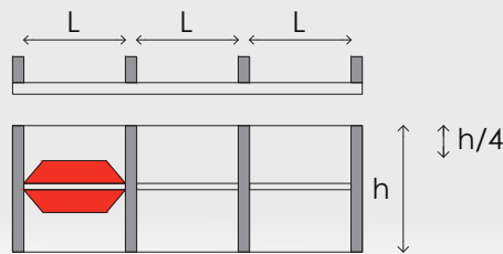
Figura 3.15. Grafico de distribución de carga para panel flexible.
