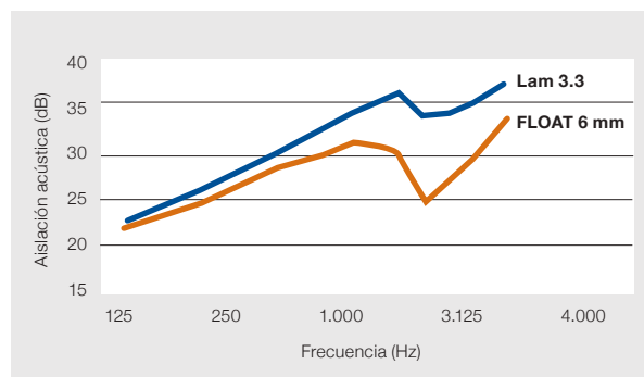
Figura 5.8. Nivel de Aislación Acústica (dB) de un cristal monolítico y laminado en función de la frecuencia (Hz).
