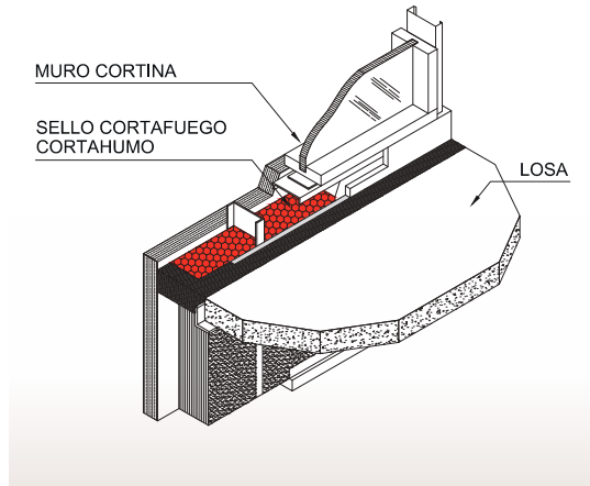
Figura 6.5. Configuración referencial certificada al fuego con detalle de materiales y componentes.
